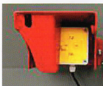
テールゲートコントロールボックス 8100/8150標準装備 7100/7150はオプションです。
